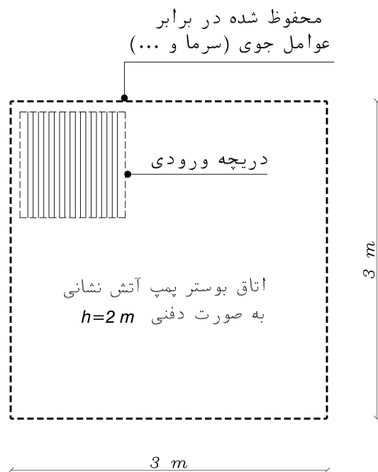
شکل پ-۶-۲- اتاق پمپ آتش‌نشانی (نمای پلان)
